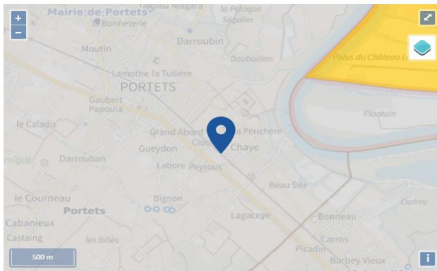
Carte de l'aléa sismique en France
