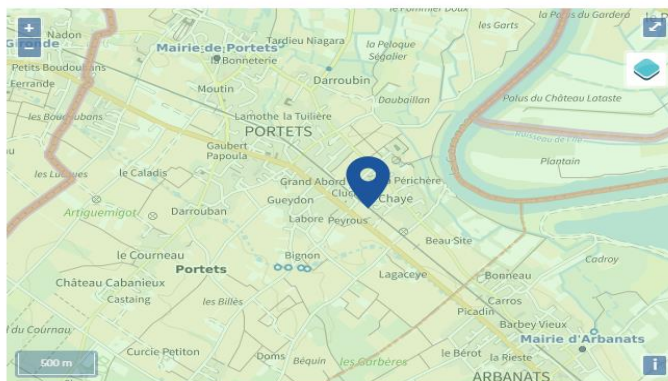
Carte du potentiel radon par commune
