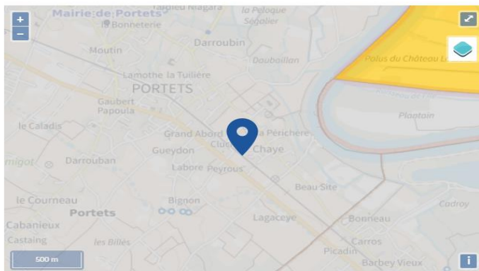
Carte de l'aléa sismique en France
